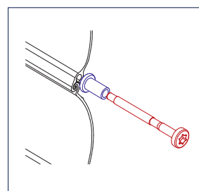
Standardausführung mit Sicherheitsarretierung (Schutz vor Herausreißen)
