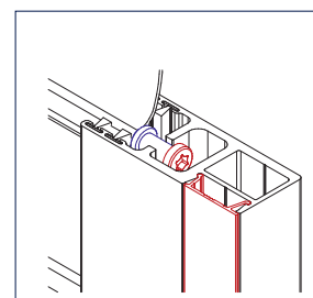
Sicherheits-Führungsschiene FSS76 76 x 32 mm gewährleistet Windwiderstandsklasse 6
